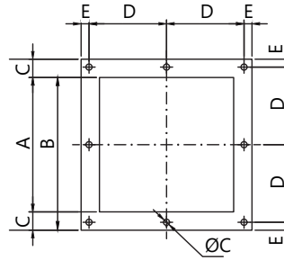
Brida cuadrada
