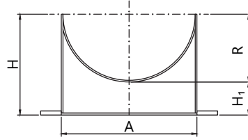
Alzado de la boca de descarga
